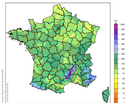
France Cumul de précipitations Octobre 2024
