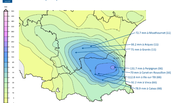
Cumuls des précipitations en 24 heures le 28 octobre 2024
