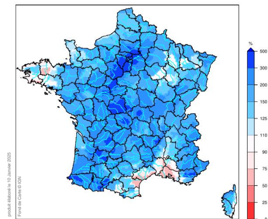
Rapport à la normale du cumul de pluies efficaces Normales calculées sur 1991 - 2020 Du 1er septembre 2024 au 31 octobre 2024
